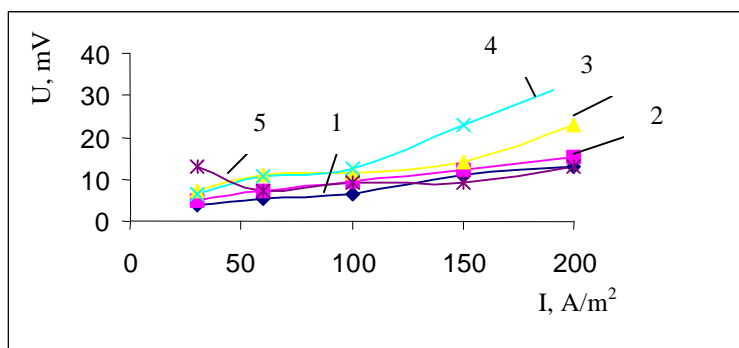
1-nji surat. Ftorid ionynyň konsentrasiýasyna baglylykda wolt-amper egrileriniň üýtgeýşi:
