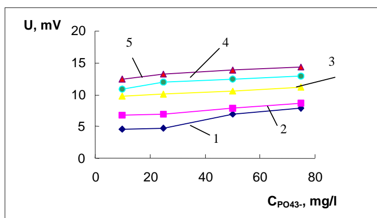
2-nji surat. Elektriki-himiki öýjükde toguň dykzlygynyň ýokarlanmagynda naprýaženiýäniň ösüşi:
