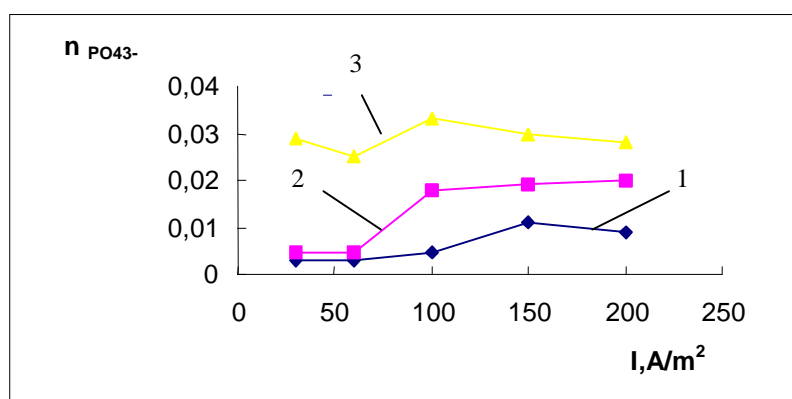
3-nji surat. Fosfat ionynyň çykymynyň toguň dykzlygyna baglylygy: 1. 25 \text{ mg/l PO}_4^{3-} ; 2. 50 \text{ mg/l PO}_4^{3-} ; 3. 75 \text{ mg/l PO}_4^{3-}
