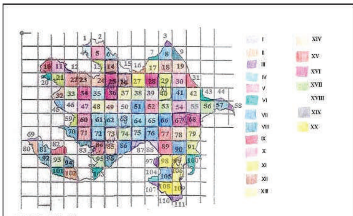
Рис. 1. Кластер районов географического соседства ландшафтов Азербайджана: по показателям среднеквадратического отклонения (а) и на основе суммарного значения (б) протяжённости географической границы
