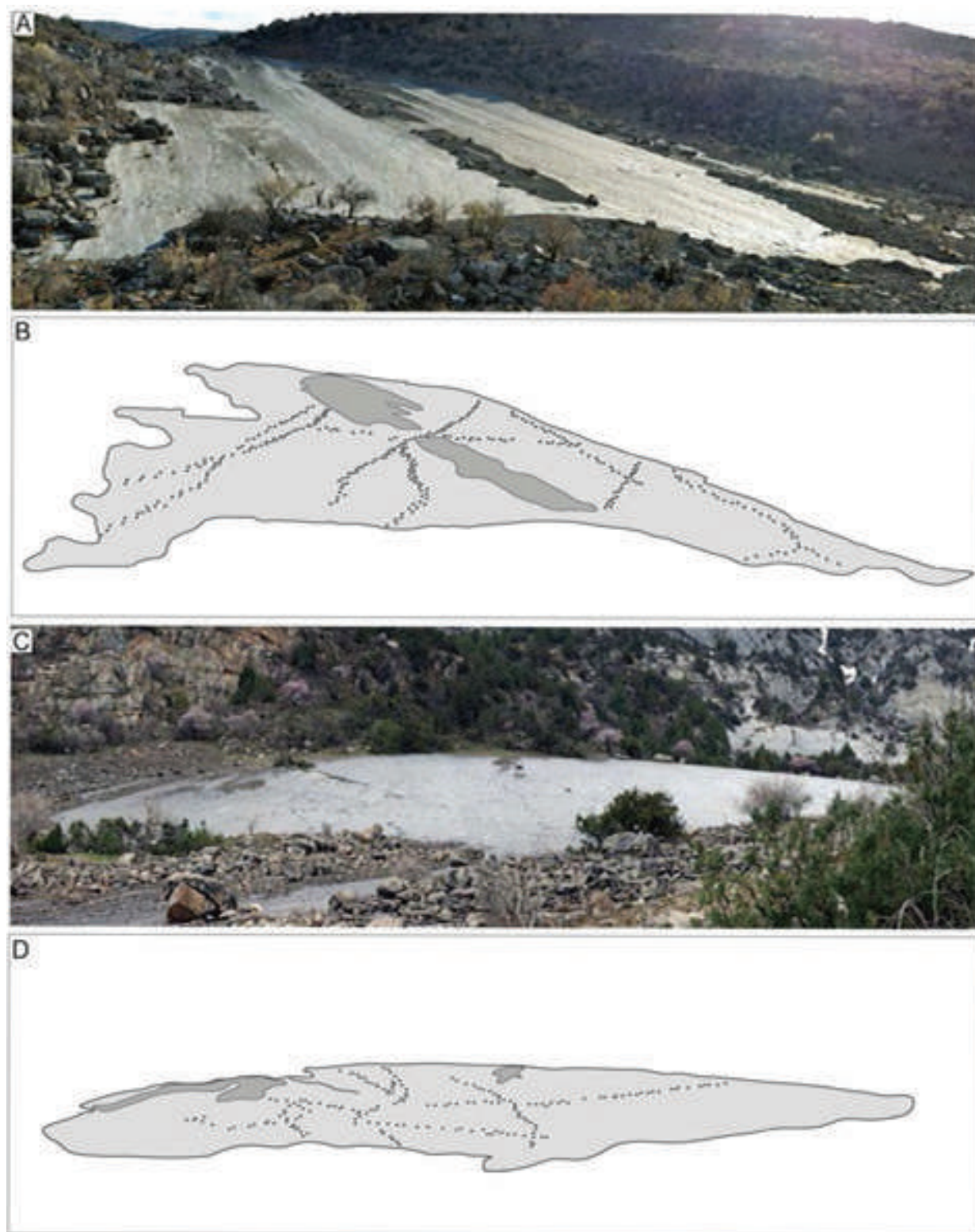
Рис.3. Фото следоносных поверхностей на Ходжапильата (А) и Акгая (С) и рисунки направления дорожек (В, D)
