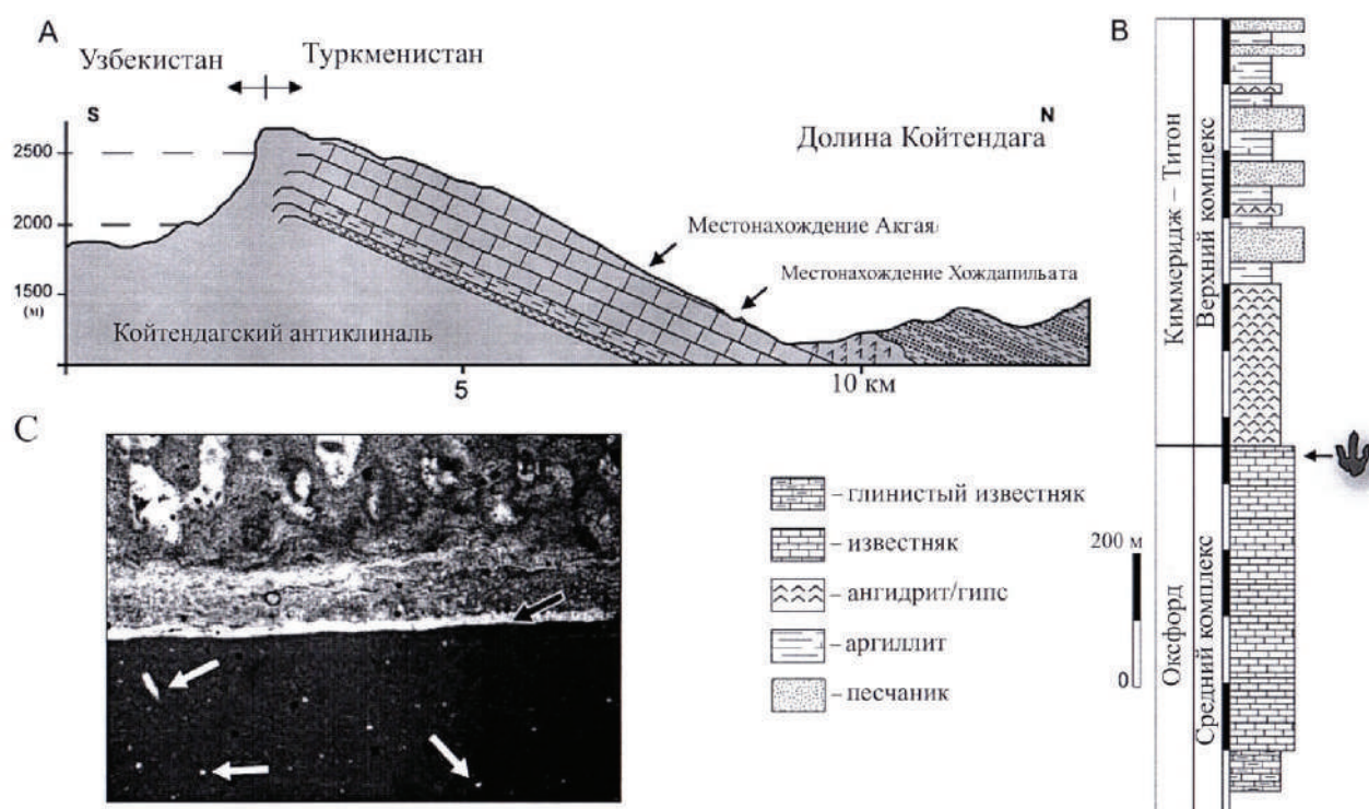
Рис. 2. Профиль койтендагской антиклинальной структуры (А); слои со следами в Ходжапильтата и Акгая, обнажающиеся приблизительно в 20 м ниже границы оксфорд – киммеридж (В); участок вытоптанной поверхности в Ходжапильтата (С), указывающий на резкое (чёрная стрелка) отделение нижнего массивного известняка от верхних органогенно-карбонатных отложений (белые стрелки указывают на обломочный материал – ракушки, остатки бентосных фораминифер и пр.)
