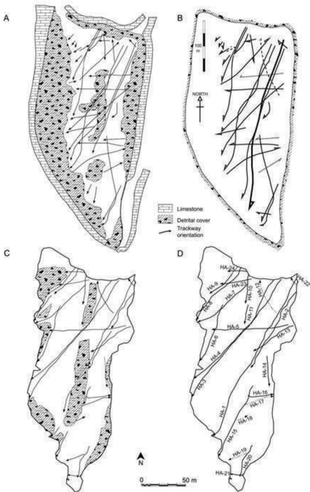
Рис. 4. Карты: местонахождение в Ходжапильата (А); составленная К.Н. Аманиязовым в 1985 г. (В); М.Г. Локли и др. в 1996 г. (С); по данным GPS (сплошные линии и пунктир – соответственно следы динозавров морфотипов 1 и 2 (D))
