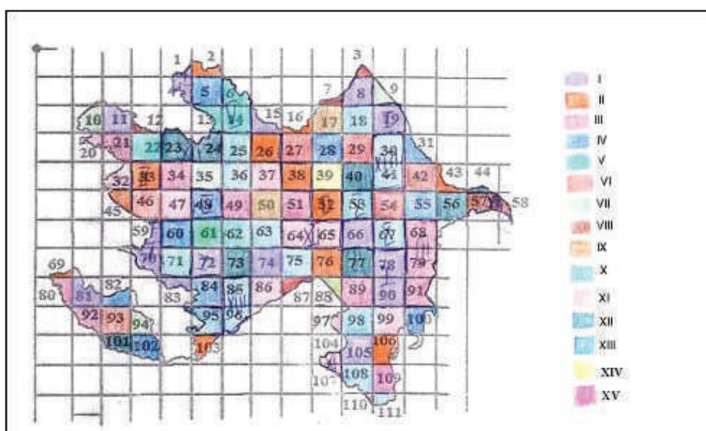
Рис. 2. Кластер районов географического соседства ландшафтов Azerbaijan на основе коэффициента вариации (а) и асимметрии (б) протяжённости границы
