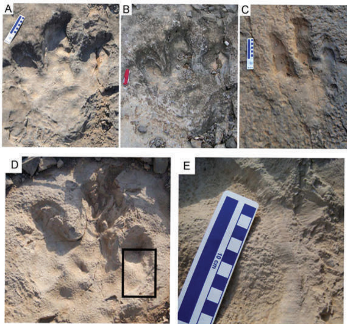
Рис. 5. Следы динозавров морфотипа 1 в Ходжапильата (А–С), следы дорожки НА-8 (D–E)
