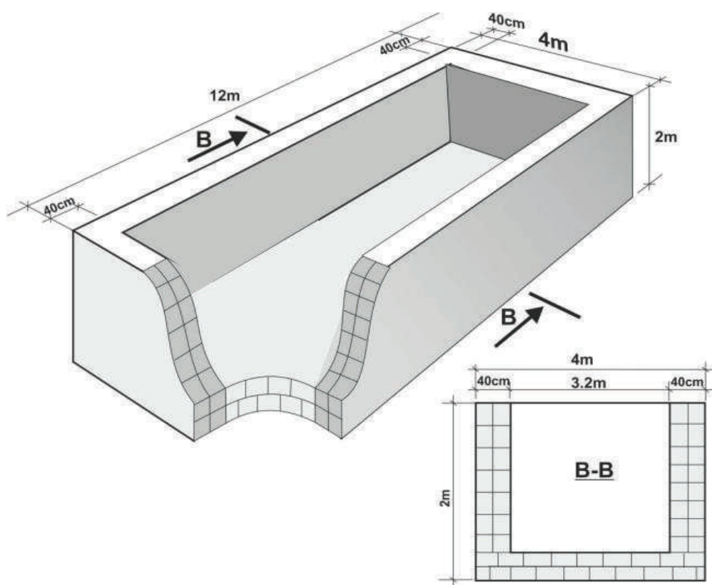
Рис. 5. Схема бассейна
