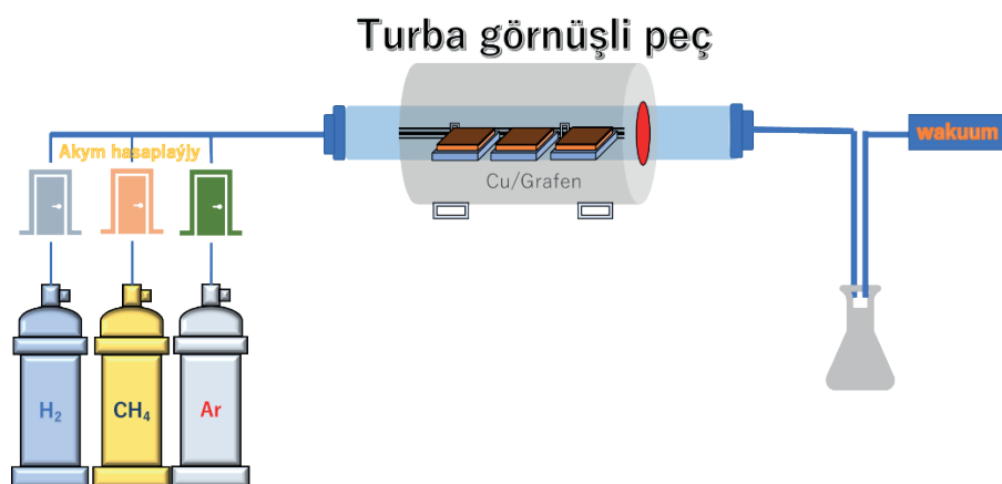
1-nji surat. Himiki bugartma-çökdürme (HBC – CVD) enjamynyň çyzgysy
