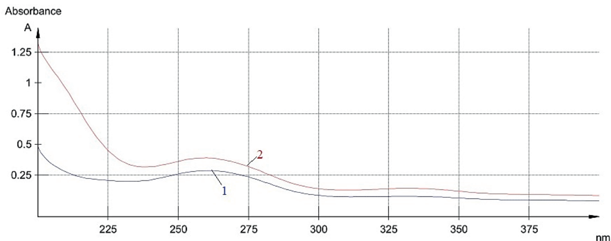
2-nji surat. Buýan köküniň galyndysy 3%-li azot kislotasynyň asetondaky ergini (2) we 3%-li trihloruksus kislotasynyň asetondaky ergini (1) bilen ekstraktsiýa edilende barlanýan B erginleriň UM – spektrleriniň deňeşdirmesi
