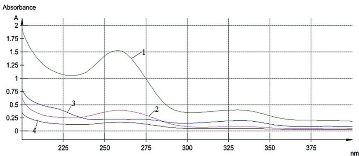
1-nji surat. Buýan kökünde (2), ondan alnan gury ekstraktynda (3), arassalanmadyk glisirizin kislotasynda (1) we buýan köküniň önümçilik galyndysynda (4) glisirizin kislotasynyň derňewinde barlanýan B erginleriň UM spektrleri
