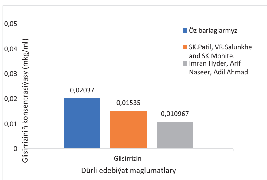
4-nji surat. Glisirriziniň mukdarynyň deňeşdirme häsiýetnamasy
