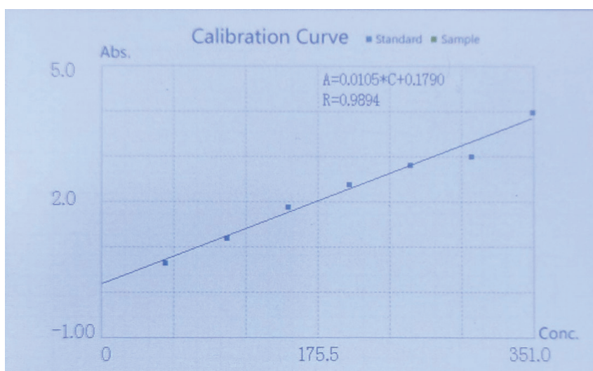
3-nji surat. Glisirriziniň standart egrisi
