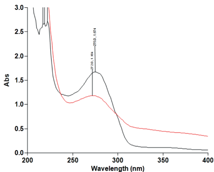
1-nji surat. Glisirriziniň spektrofotometr barlagynyň netijesi
