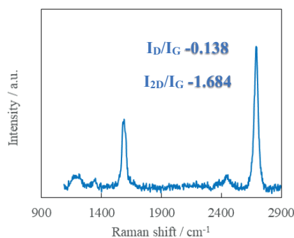
2-nji surat. Sintezlenen grafeniň Raman spektrometriýasynyň netijesi
